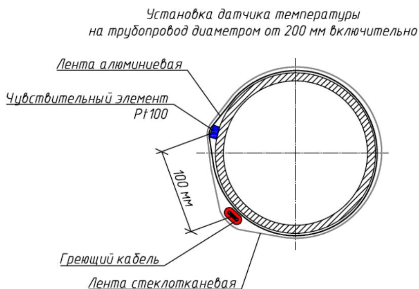
Рисунок 5 – Установка датчика температуры на трубопроводе
