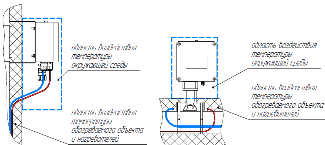
Рисунок 1 – Части термостата, отличающиеся температурой воздействия
