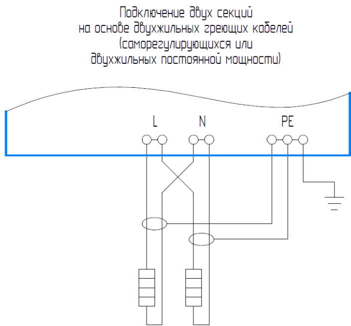
Варианты схемы подключения нагрузки к термостату ТСВ-1-М-Х
