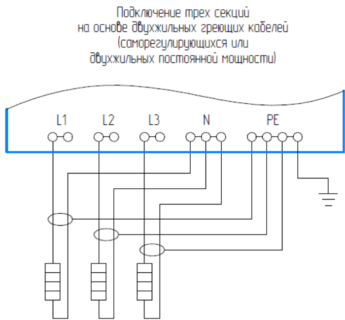
Варианты схемы подключения нагрузки к термостату ТСВ-3-Д-Х
