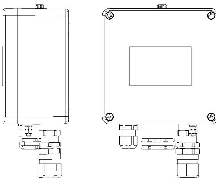
Рисунок 2 - Общий вид
