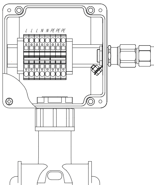
КСТ-КС-П-Л(6)/3;N(6)/2;PE(6)/3-П-В: НПС(7,5x5,5-13,8x6,6)/1-D:БКО(9-25)/1
